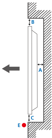
图 1.2 侧视图
