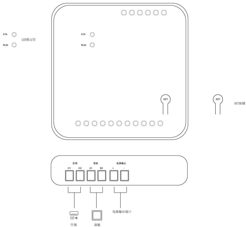
AGW05RT空调网关接线图
