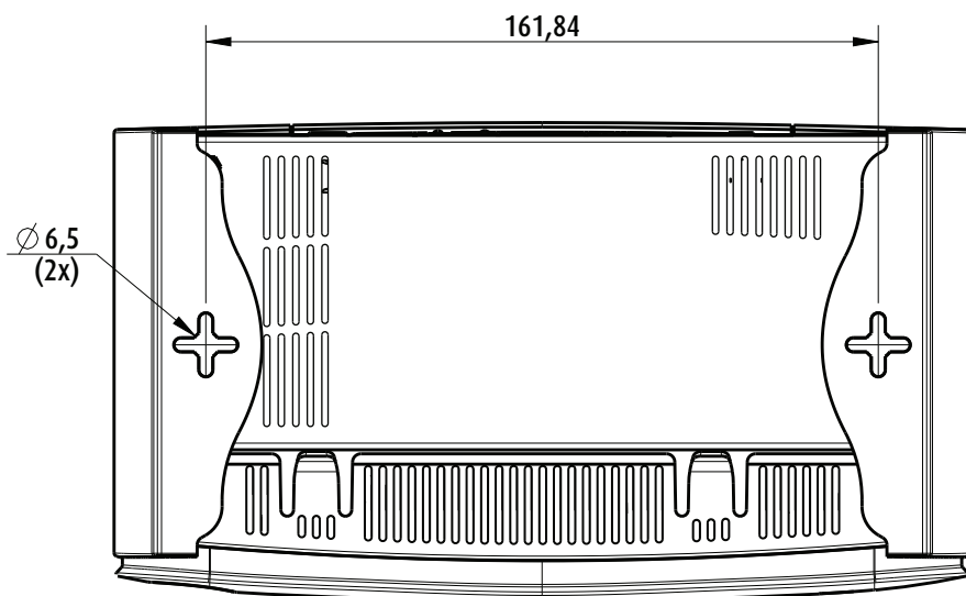
图像 4-1: 安装孔
