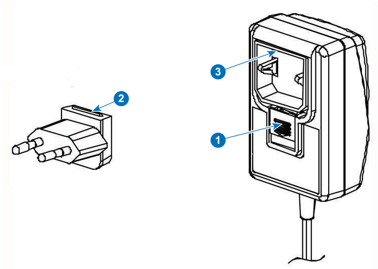
图像 4-4: 安装适配器
