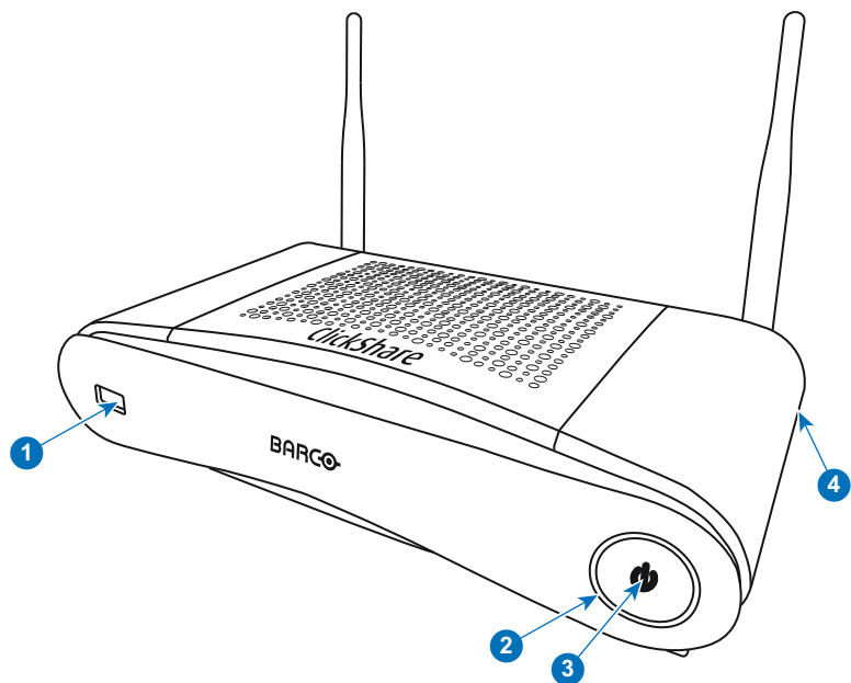
图像 2-2: Base Unit 的前面板
