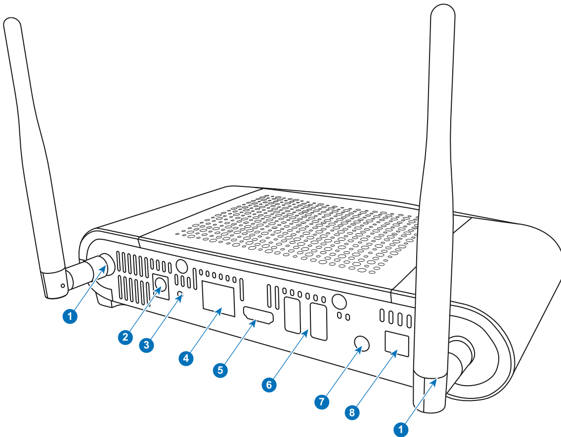
图像 2-3: Base Unit 的后面
